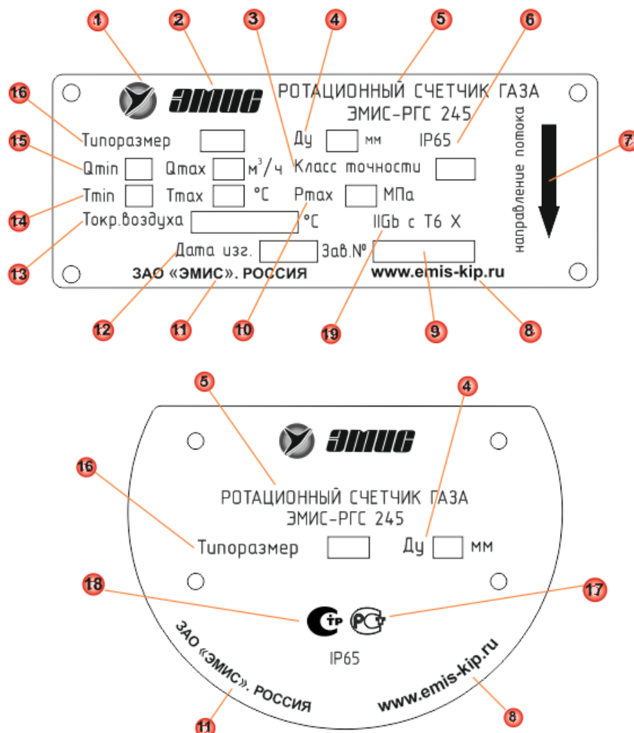
Рисунок 1.8 – Вид верхнего и переднего шильда счетчика
