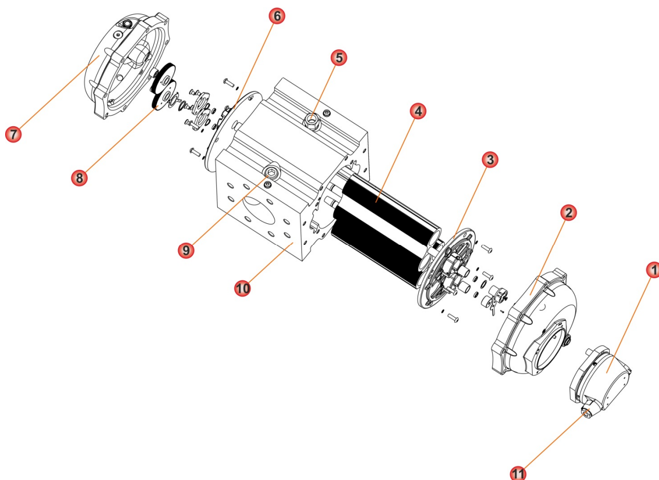
Рисунок Б.1 – Конструкция счетчика
