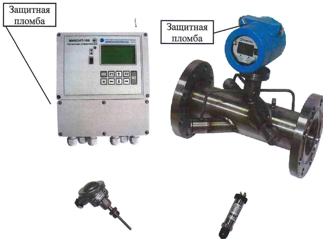
Рисунок 2 — Счётчик газа ультразвуковой СГУ.2
