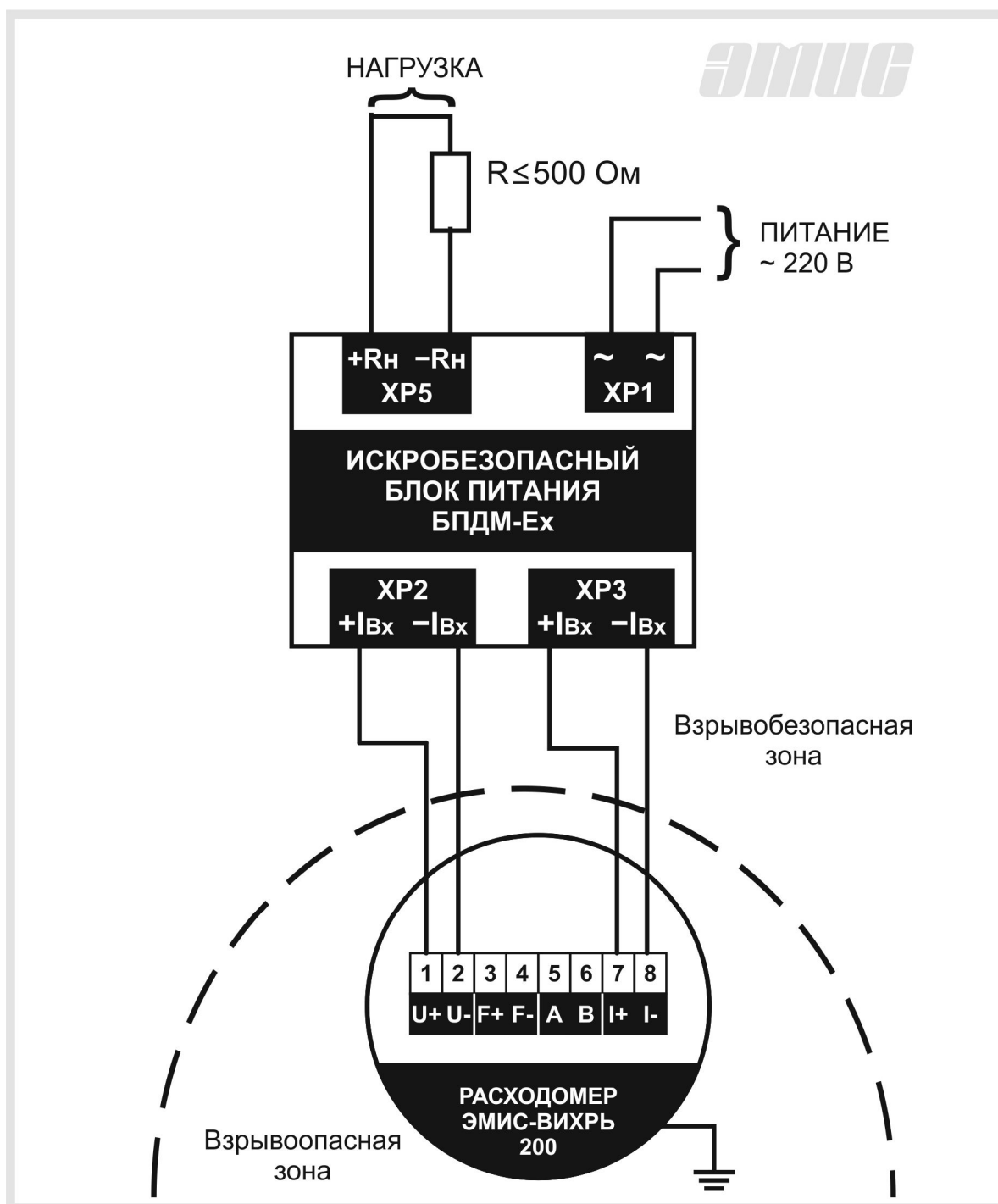
Рисунок Б.9 – Схема подключения преобразователей взрывозащищенного исполнения ExB и ExC к искробезопасному блоку питания с использованием токового выходного сигнала на примере блока питания БПДМ-Ex
