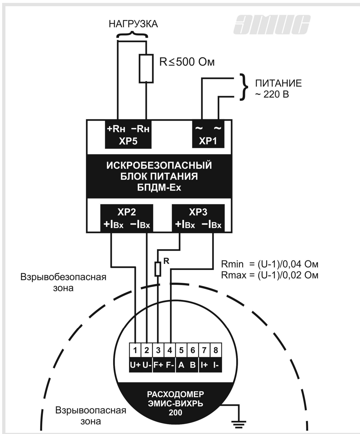
Рисунок Б.8 – Схема подключения преобразователей взрывозащищенного исполнения ExB и ExC к искробезопасному блоку питания с использованием частотного выходного сигнала на примере блока питания БПДМ-Ex
