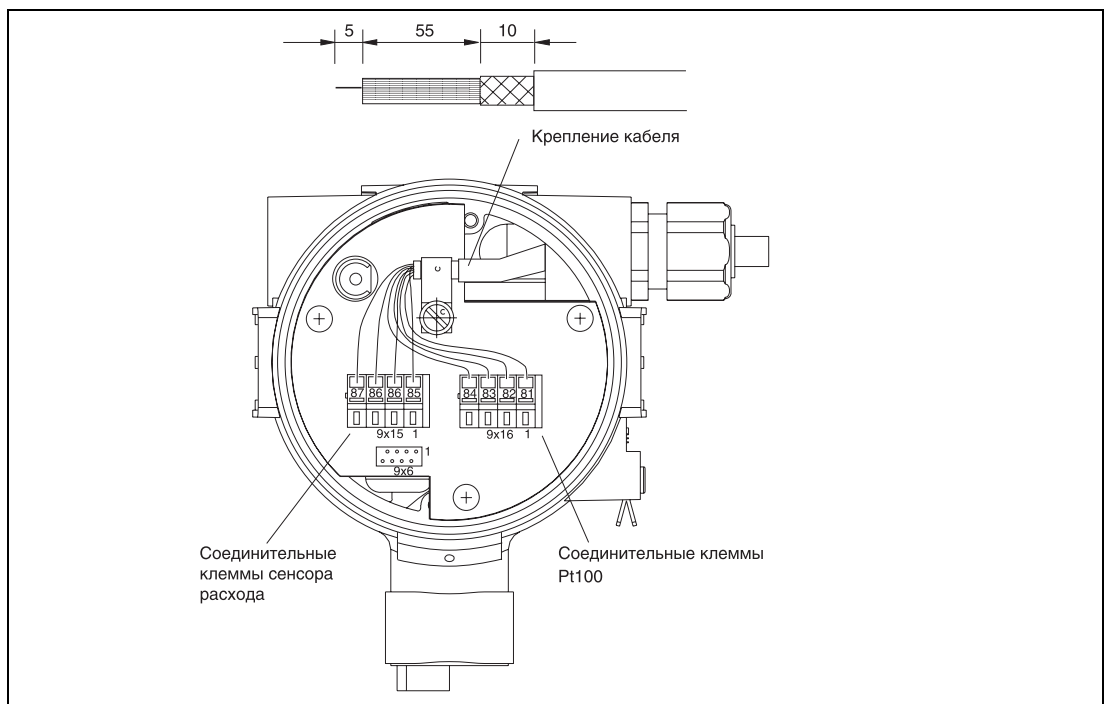
Рис. 30: Клеммный блок первичного преобразователя вихревого расходомера.
