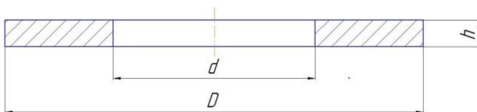
Рисунок А.4 – Размеры фланцевых прокладок
