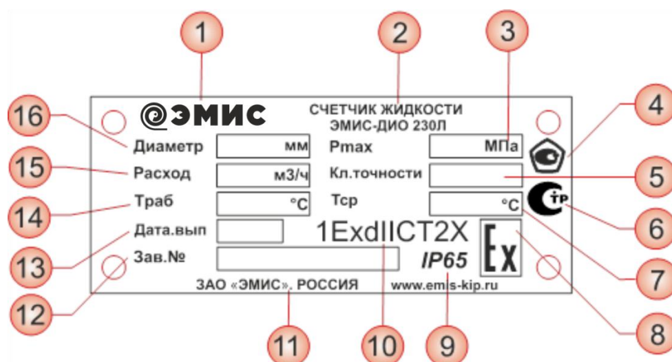
Рисунок 1.5 - Табличка счетчика
