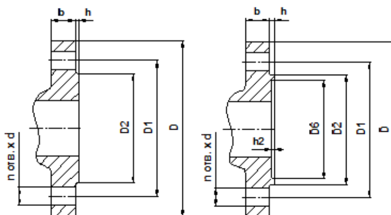
Рисунок А.2 – Присоединительные размеры фланцев
