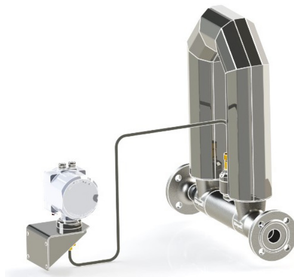
Общий вид Счетчиков-расходомеров массовых Штрай-Масс с выносным ЭБП
