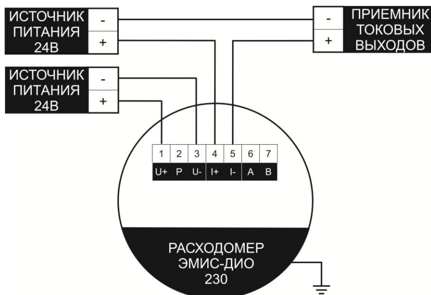
Рисунок Г.4 – Схема подключения, токовому выходному сигналу
