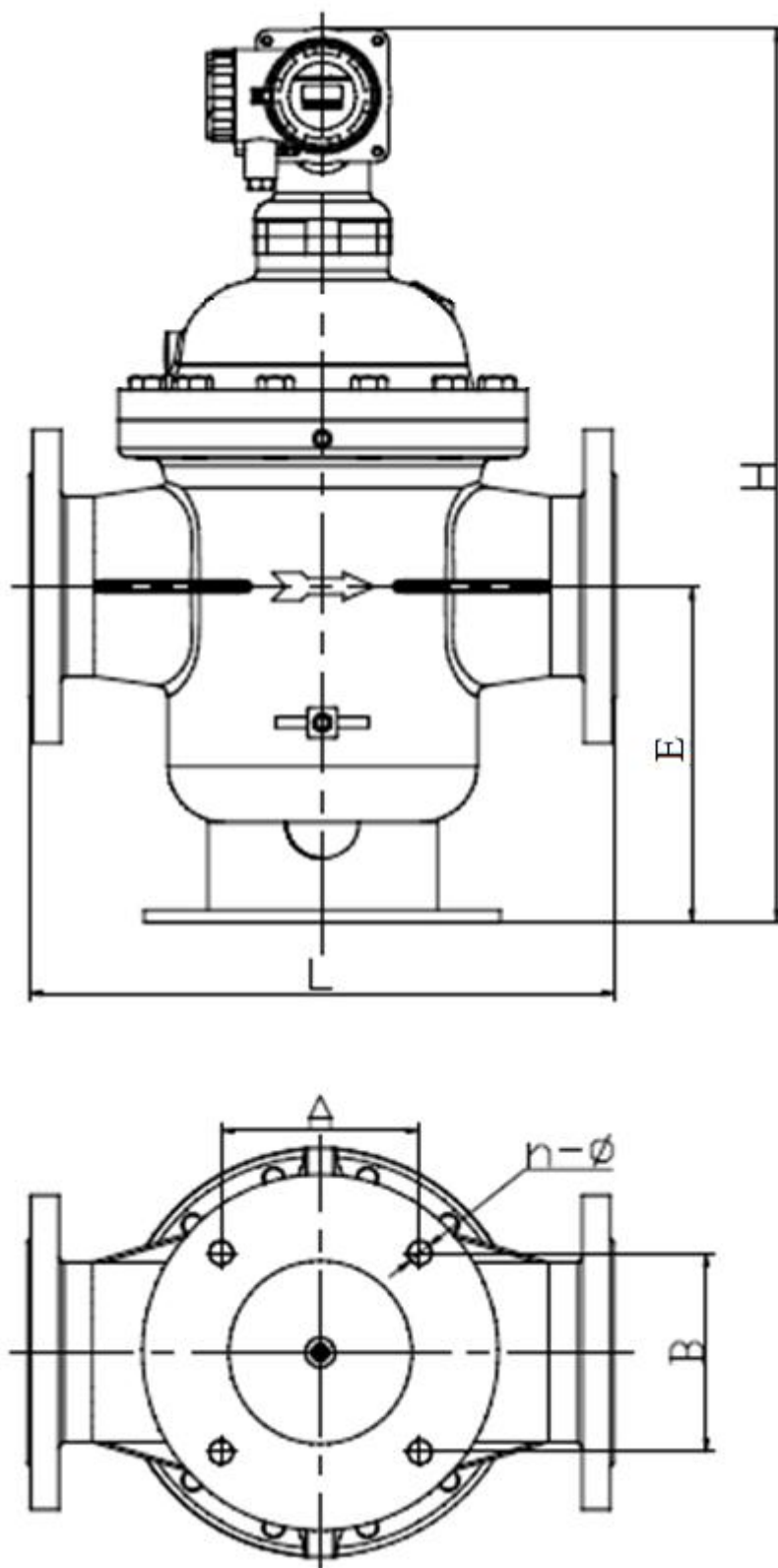
Рисунок А.4 – Внешний вид счетчика Ду = 100-150 мм
